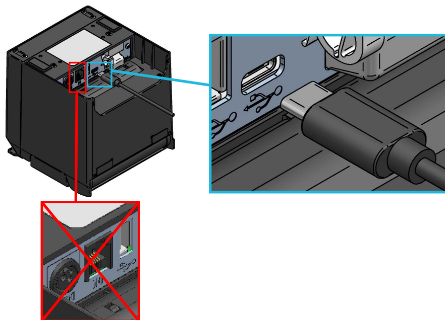
Figura 12-3 Conexión de la impresora y del cable USB-C
