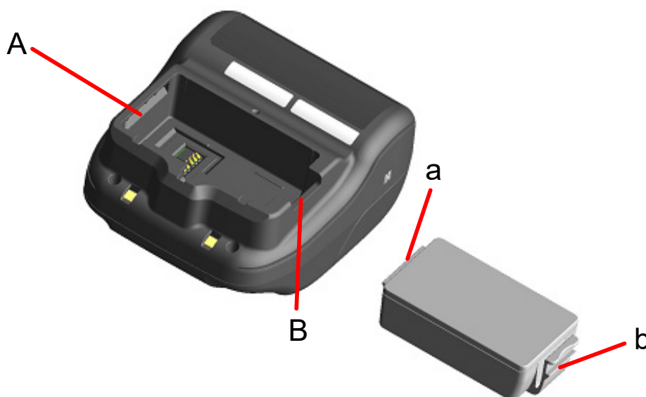
Figura 8-1 Orientação da bateria
