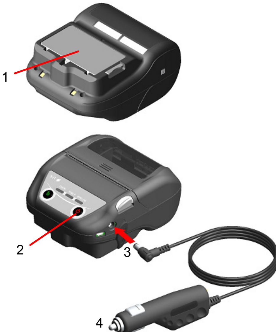
Figura 16-2 Carregamento no modo de carregamento ligado por carregador para automóvel
