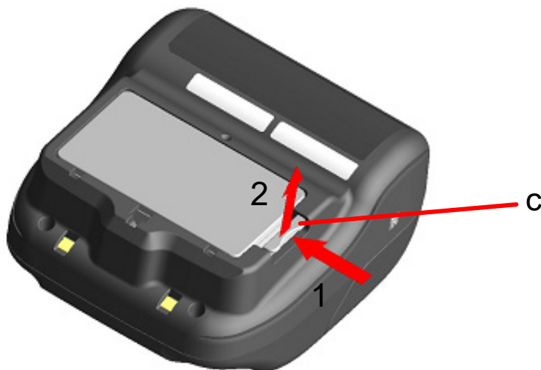
Figura 8-4 Remoção da bateria
