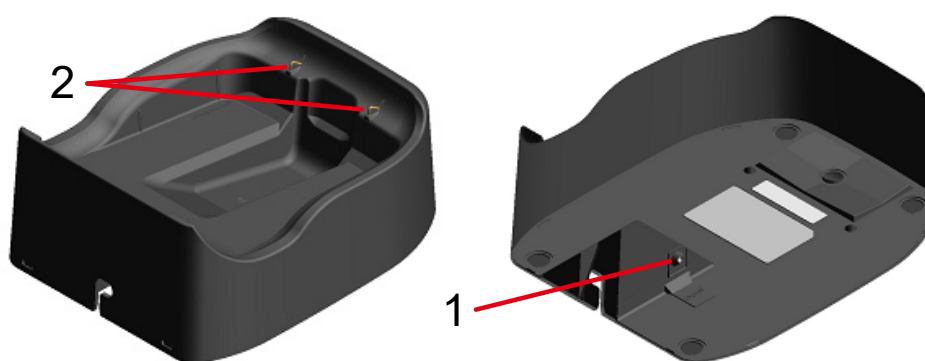
Figura 15-1 Cada peça da base (CDL-B02K-1)
