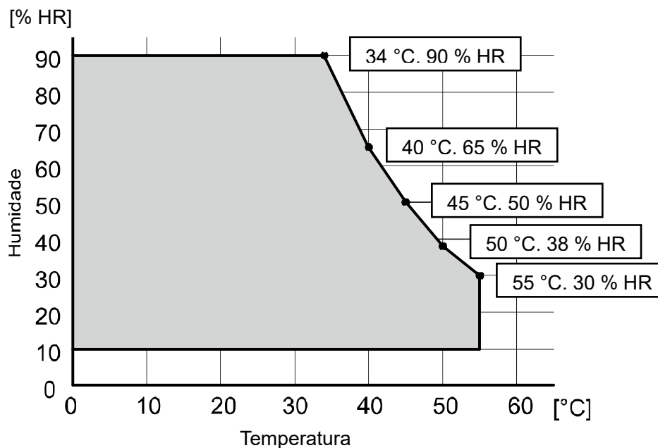
Figura 20-1 Temperatura de funcionamento e intervalo de humidade (impressão)
