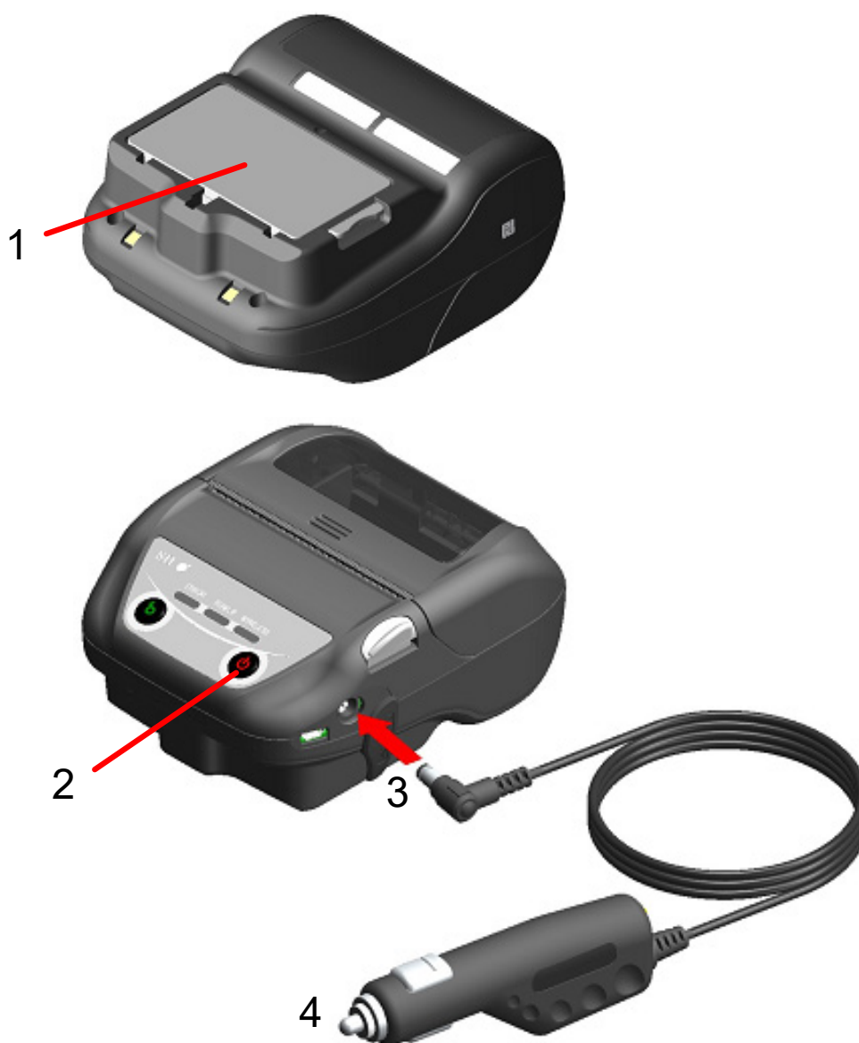
図 16-2 カーチャージャによるパワーオン充電モードでの充電
