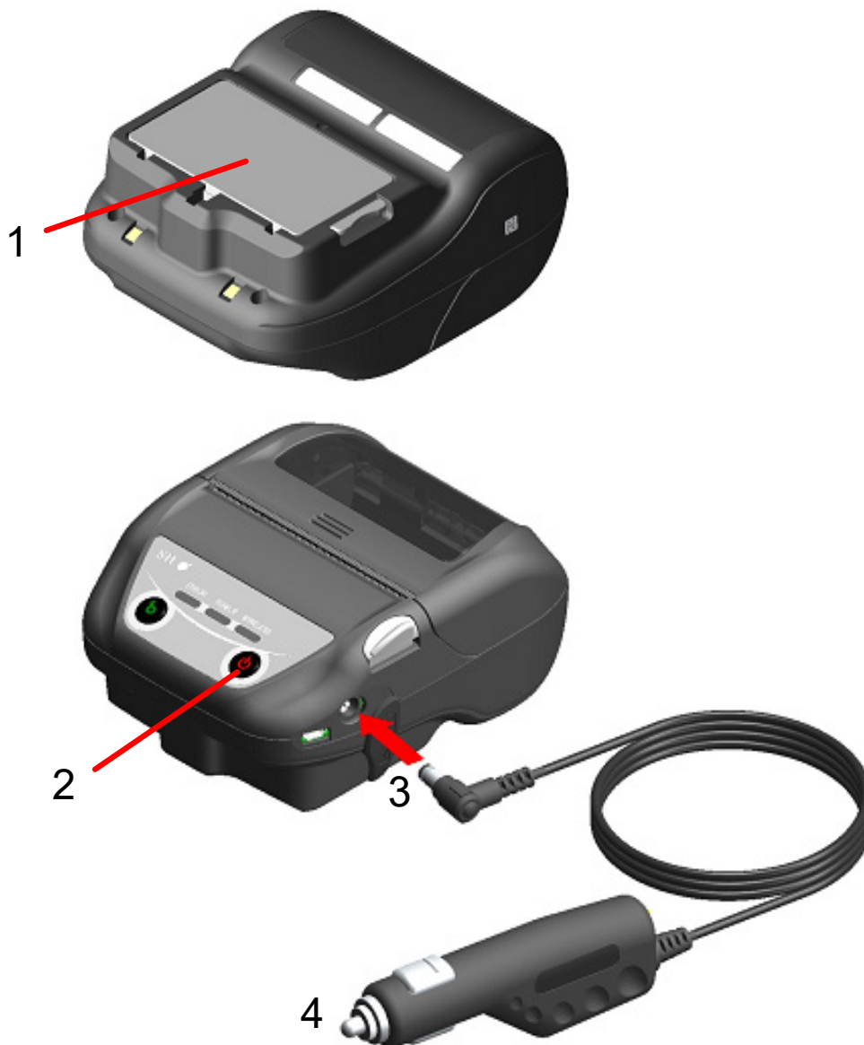
Figura 16-2 Modalità di carica con stampante accesa mediante caricatore per auto
