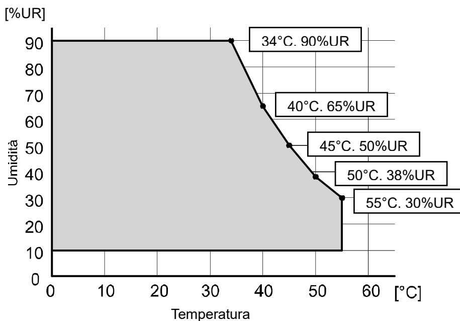
Figura 20-1 Intervallo di temperatura operativa e umidità (durante la stampa)
