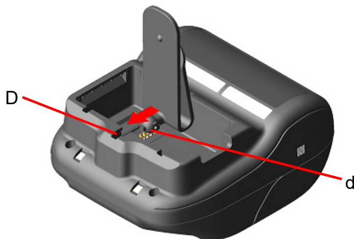
Figura 13-1 Installazione della clip da cintura (1)
