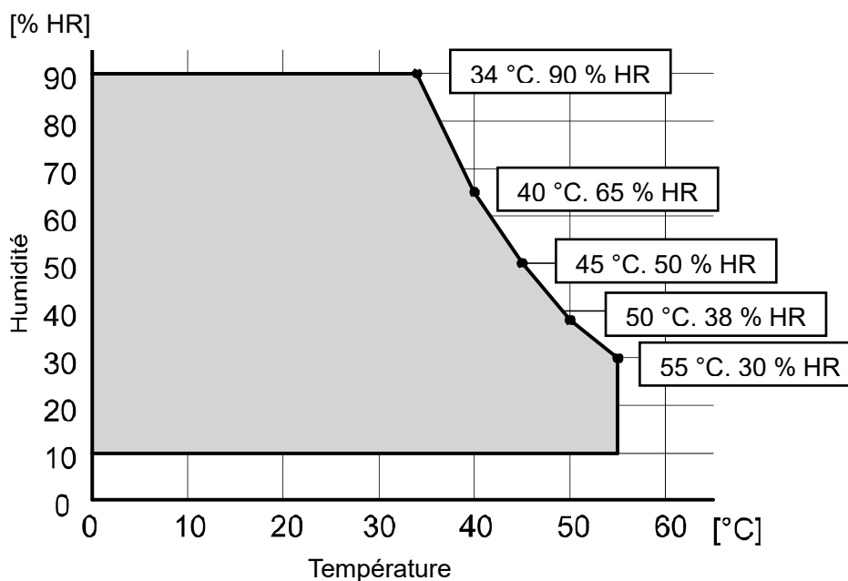
Illustration 20-1 Température de fonctionnement et gamme d'humidité (impression)
