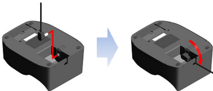
Illustration 15-2 Connexion de la station d'accueil avec l'adaptateur c.a.
