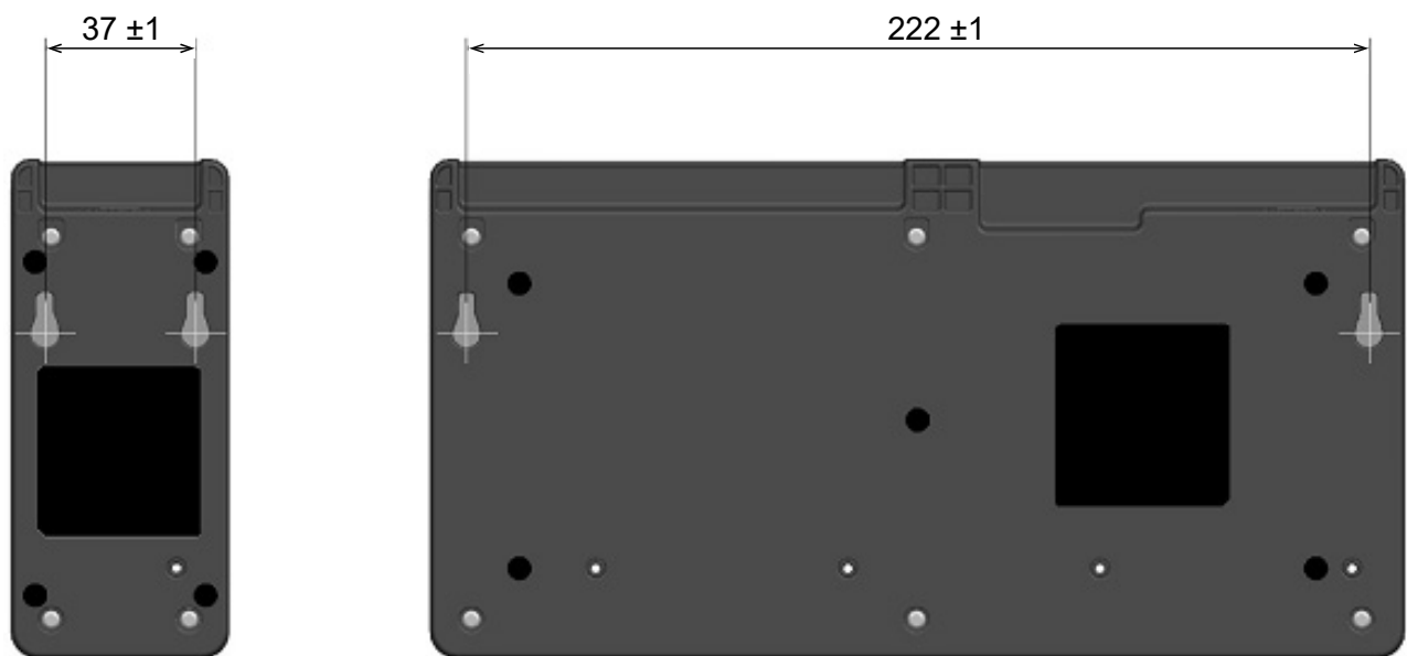
Illustration 17-8 Partie inférieure du chargeur de batterie
