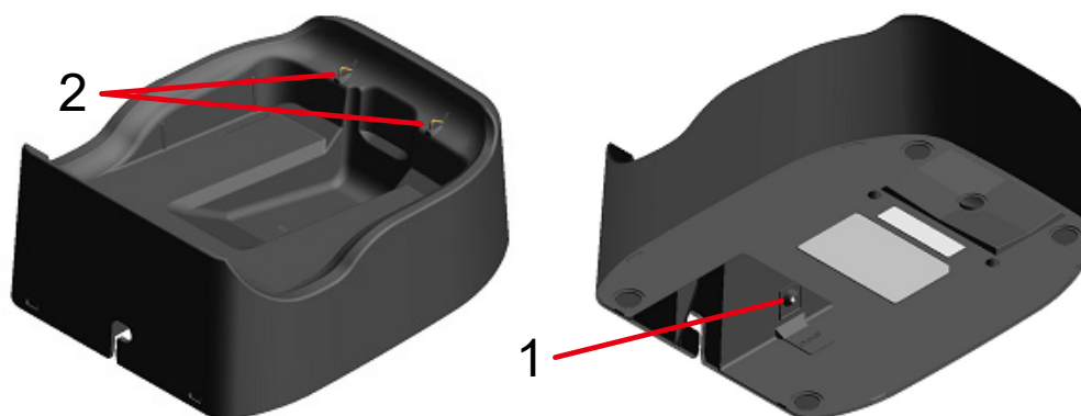
Illustration 15-1 Composants de la station d'accueil (CDL-B02K-1)
