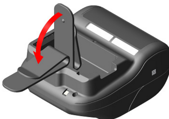
Illustration 13-2 Montage du clip de ceinture (2)
