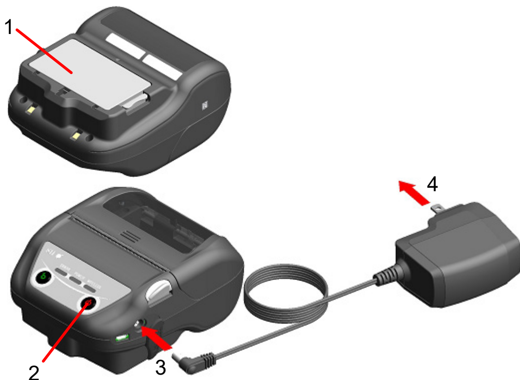
Illustration 14-1 Chargement en mode de chargement sous tension avec l'adaptateur c.a
